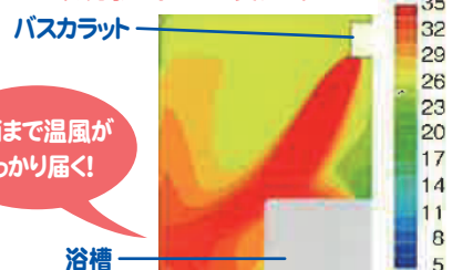
暖房強時の温度分布図
